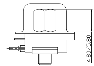
鉚合鎖螺絲型
