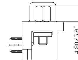
鉚合鎖螺絲型
