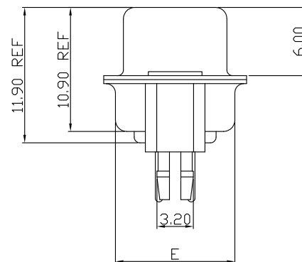
鉗合型
